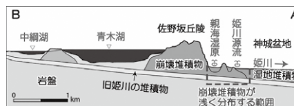
図2 A-B断面(縦の縮尺は横の4倍)
