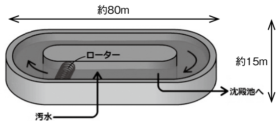
オキシデーションディッチ法の模式図。ローターが回転することで水をかき混ぜて酸素を水槽に送り込み、微生物の活動を促進する。スケールは白馬のもの。水深3m程度。(畜産環境技術研究所HPより引用。一部編集)
