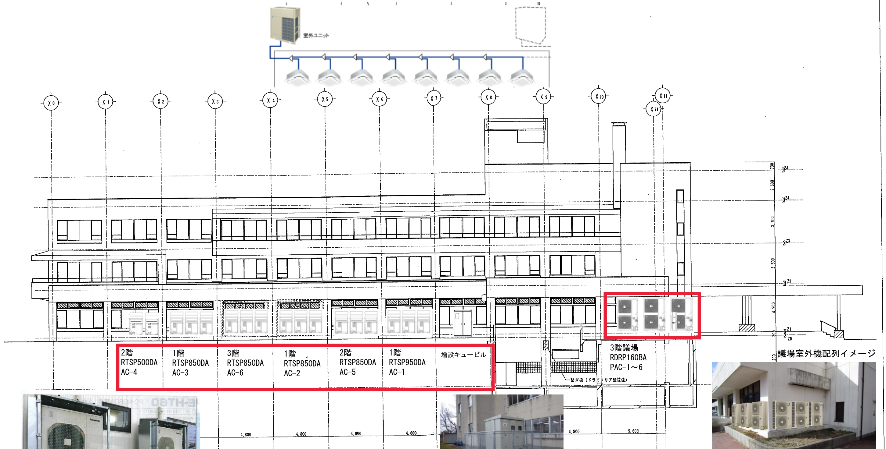
南立面図 S=1/100
