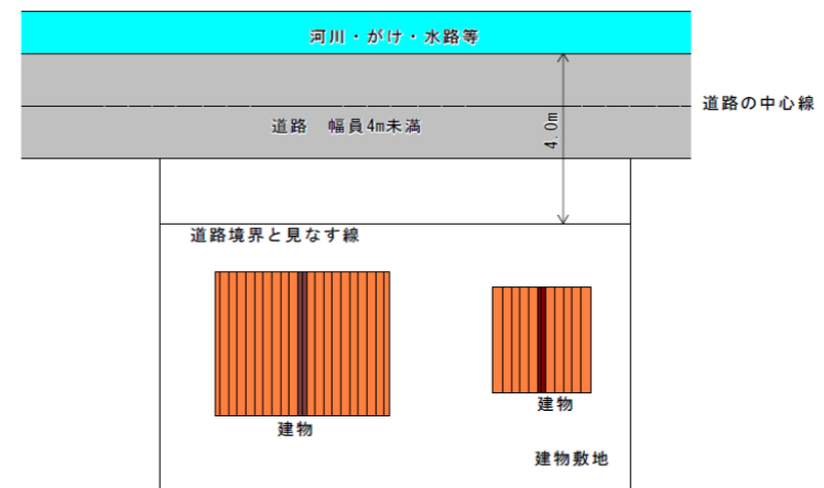
図 建築基準法第42条第2項による道路境界の考え方
